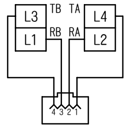
回路図
