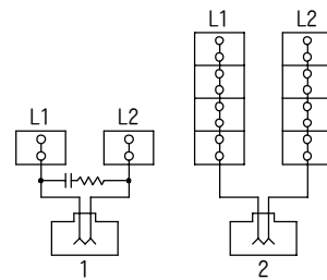
回路図
