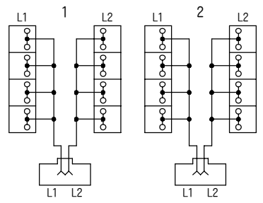
回路図
