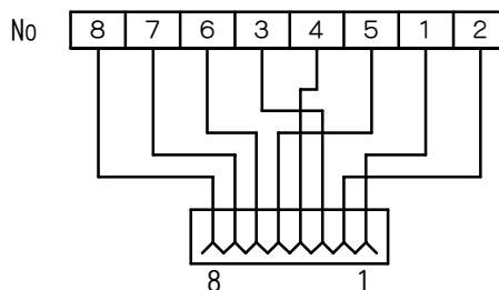
回路図
