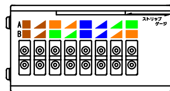
LAN配線用「コード」表示図
