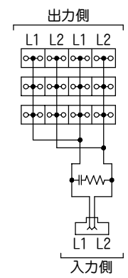
回路図
