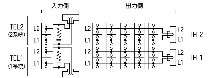
回路図
