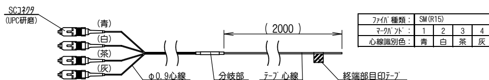
4心SC光F0心線 外観図
