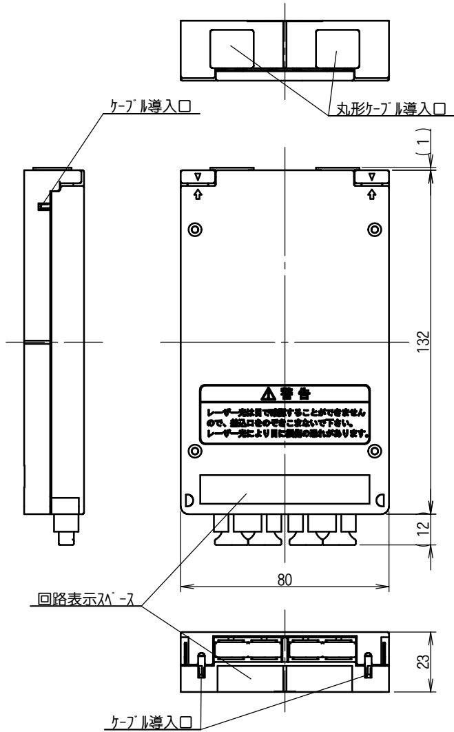
2心SC光F0心線 外観図
