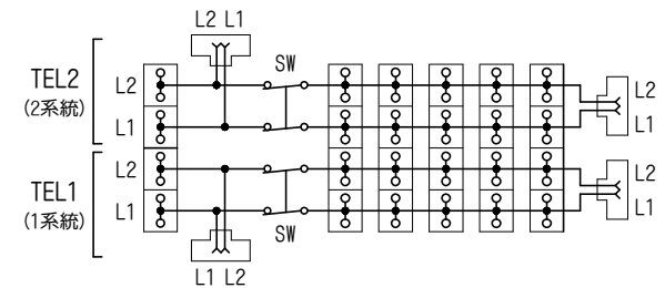
回路図
