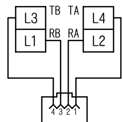
回路図
