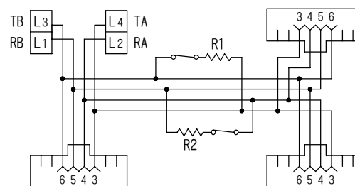
回路図
