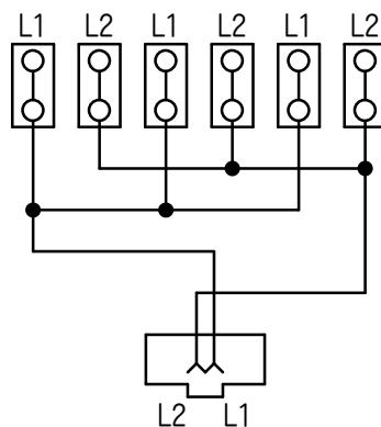
回路図
