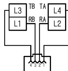
回路図
