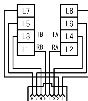
回路図
