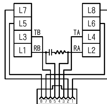
回路図
