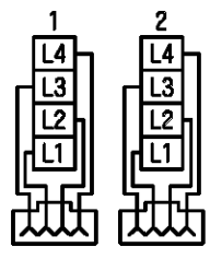
回路図
