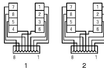
回路図
