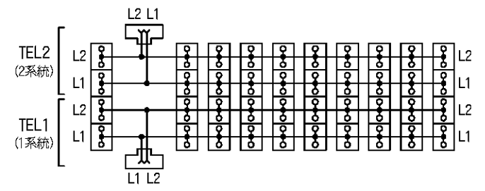
回路図
