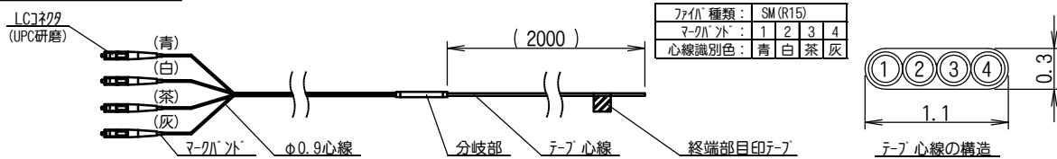
4心LC光F0心線 外觀図
