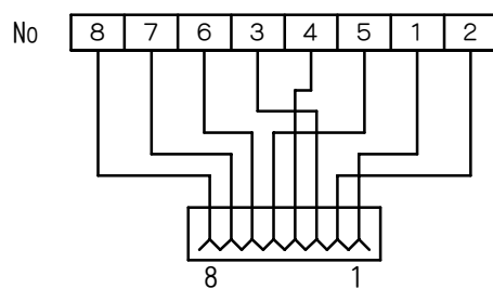
回路図
