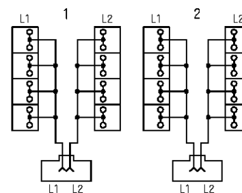
回路図
